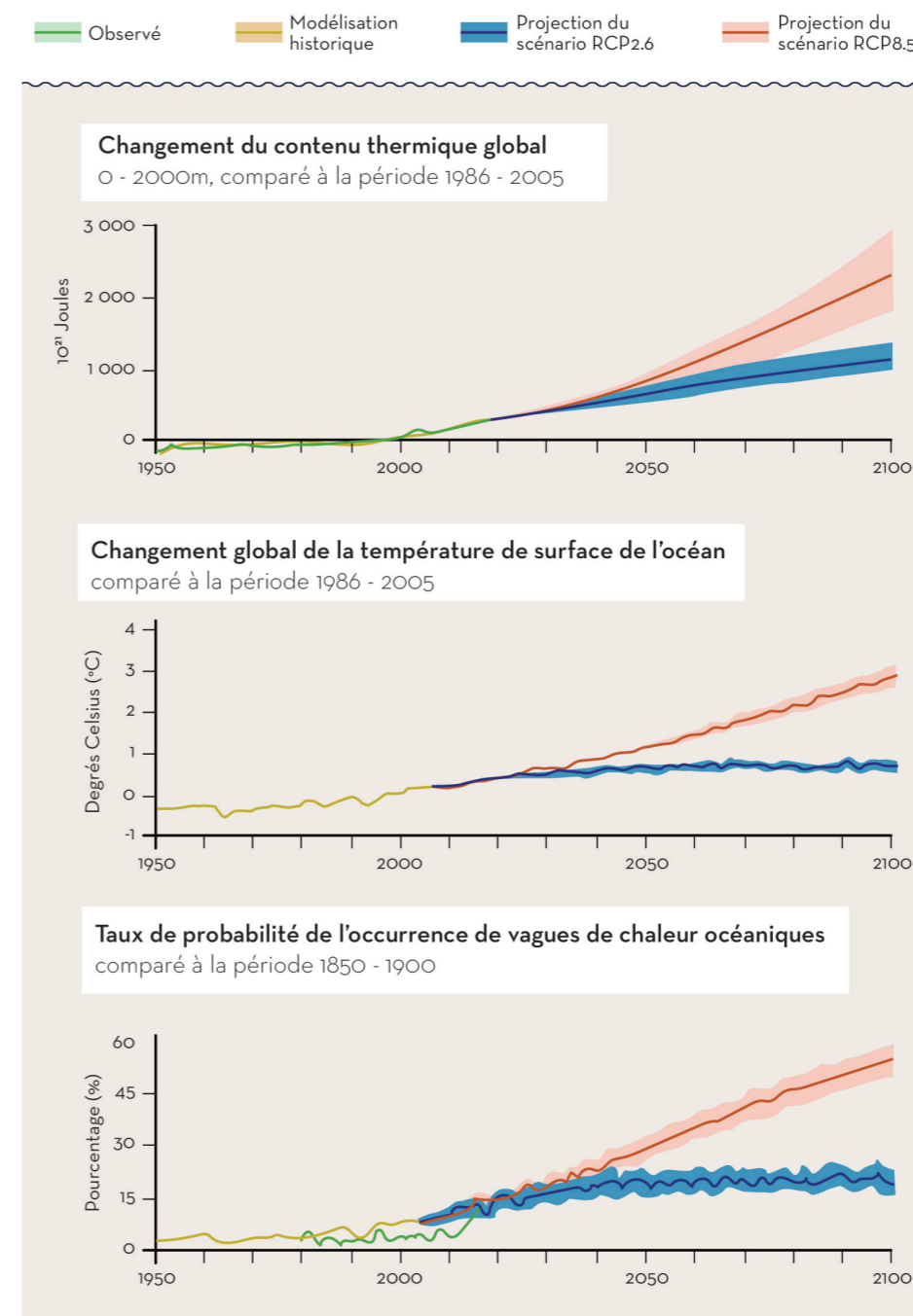
Figure 2 : Changements affectant l'océan: observations et projections concernant le contenu thermique et la probabilité de l'occurrence de vagues de chaleur selon les scénarios d'émissions basses (RCP2.6) et hautes (RCP8.5). Source: IPCC, SROCC, 2019. SPM
